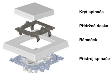
Obr. 10: Sestavování spínače Levit® s krytem a rámečkem
