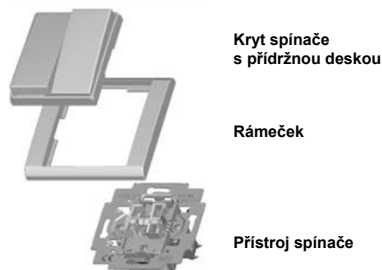
Obr. 4: Sestavování spínače s krytem a rámečkem
